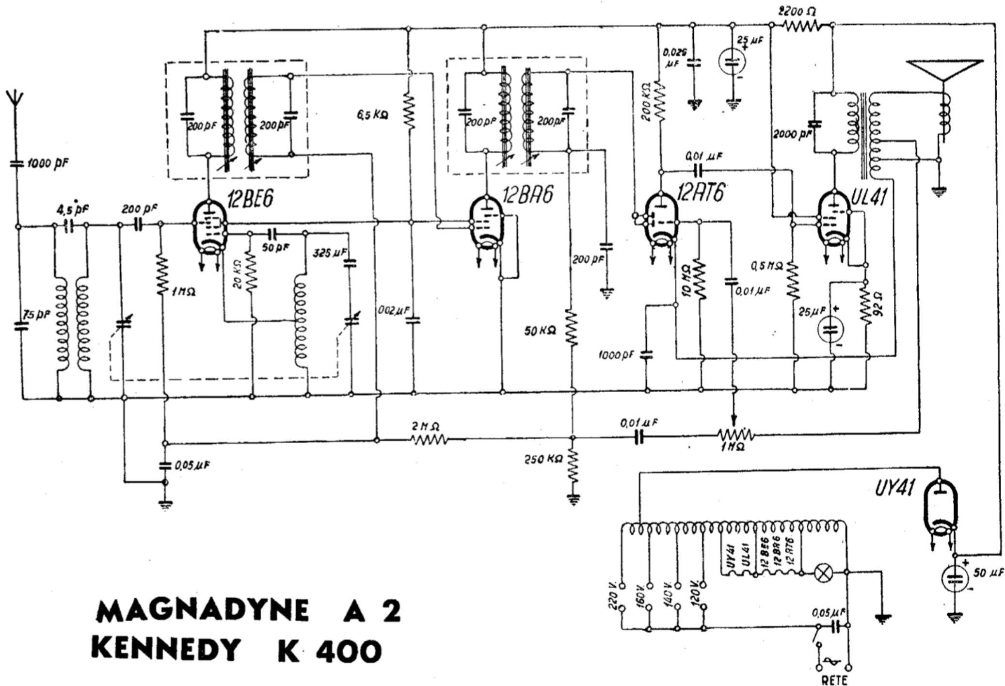
MAGNADYNE RADIO - Modd. MAGNADYNE A 2 e KENNEDY K 400. Una sola gamma onde medie. Lo stadio finale è provvisto di controreazione. Potenza di uscita 3 watt.
